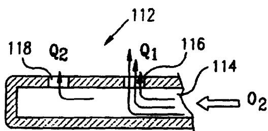
FIG. 9A PRIOR ART
