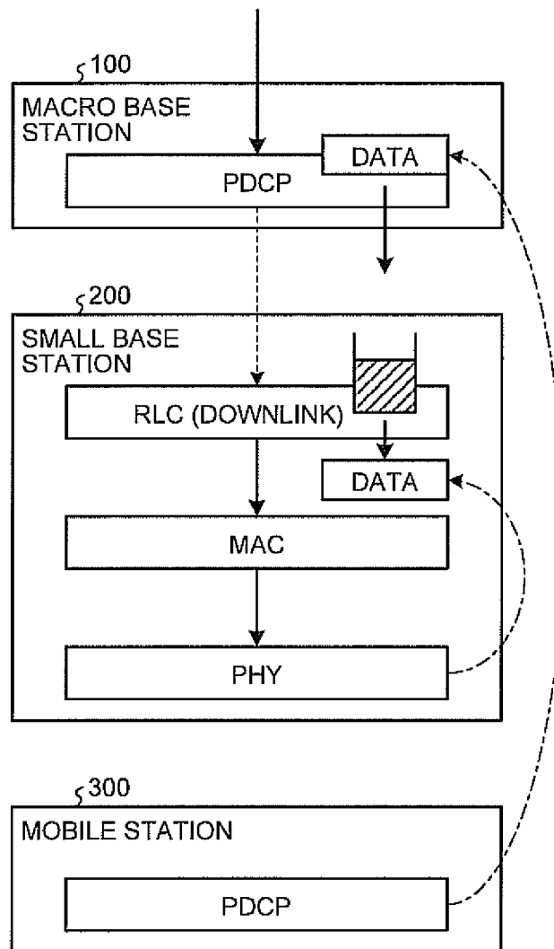
FIG.11B
