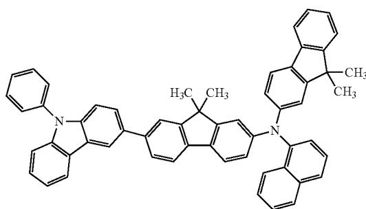
&lt;Compound 4&gt;
