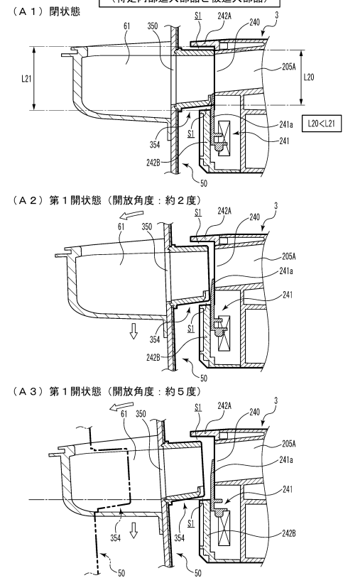
【図13-49】 払出通路 (特定内部進入部品と被進入部品)
