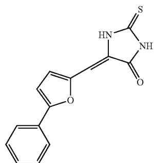
Compound E15
