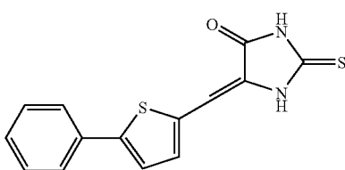
Compound E16
