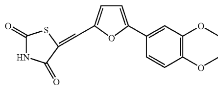
Compound F1
