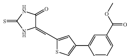
Compound E14
