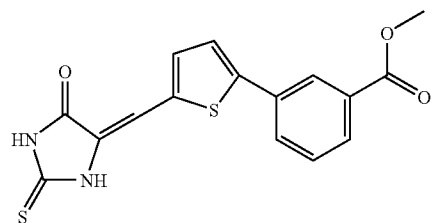
Compound E11
