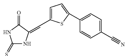
Compound E10
