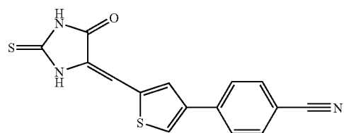
Compound E13
