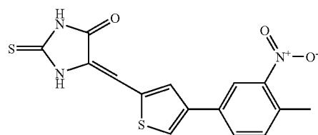
Compound E12
