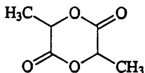
L-Lactide
