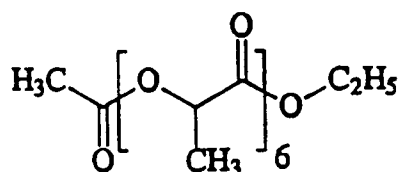
Ac-(PLA) 6 -OEt
