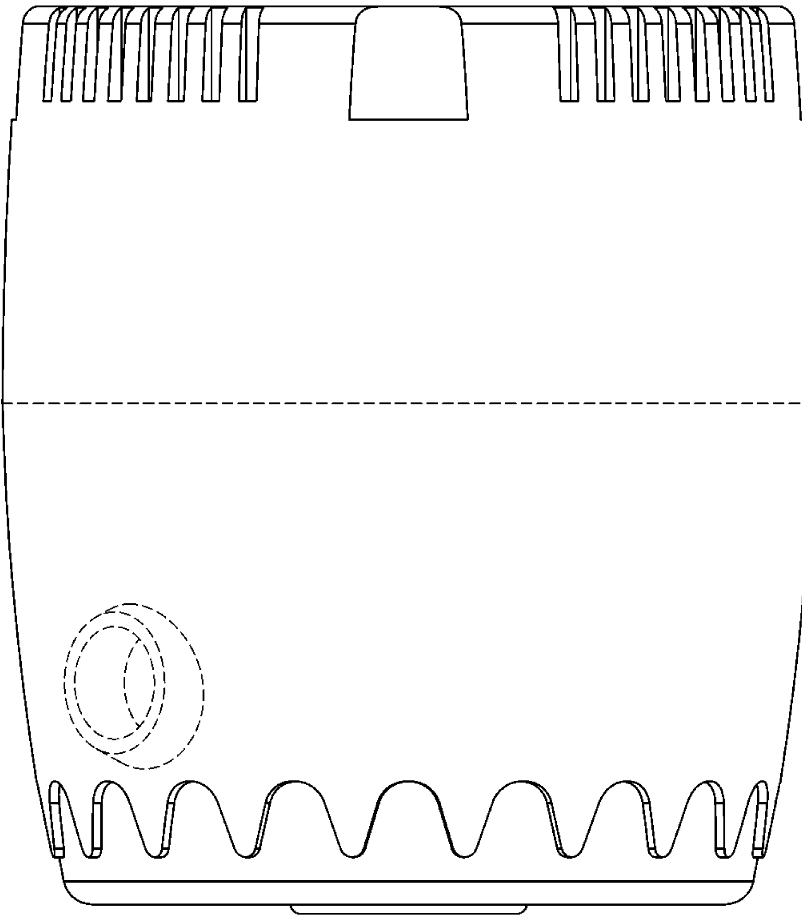
後視圖
