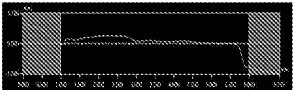
거칠기 곡선
