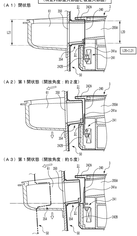
【図13-49】 私出通路 (特定内部進入部品と被進入部品)
