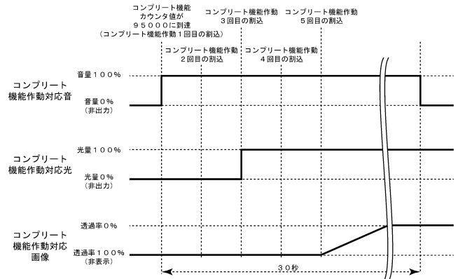
コンプリート機能動作時の出力タイミング
