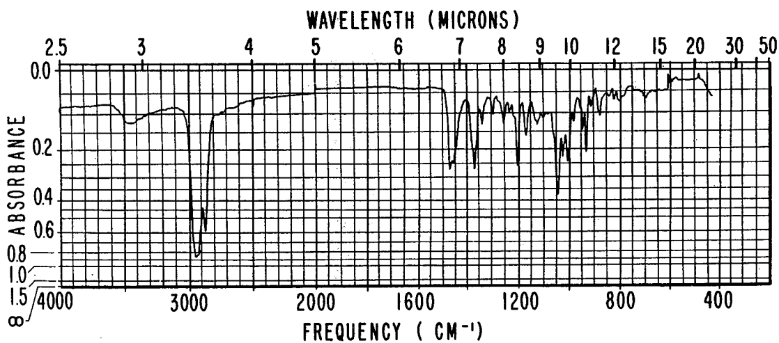
IR SPECTRUM FOR EXAMPLE II
