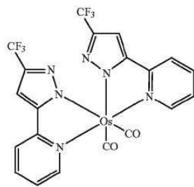
Os(fppz) 2 (CO) 2
