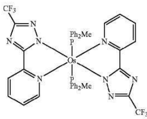
Os(fptz) 2 (PPh 2 Me) 2
