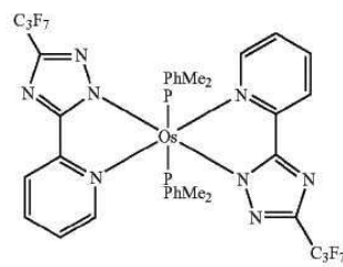
Os(hptz) 2 (PPhMe) 2
