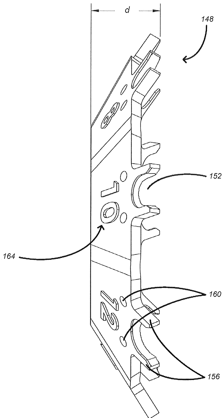
FIG. 7C
