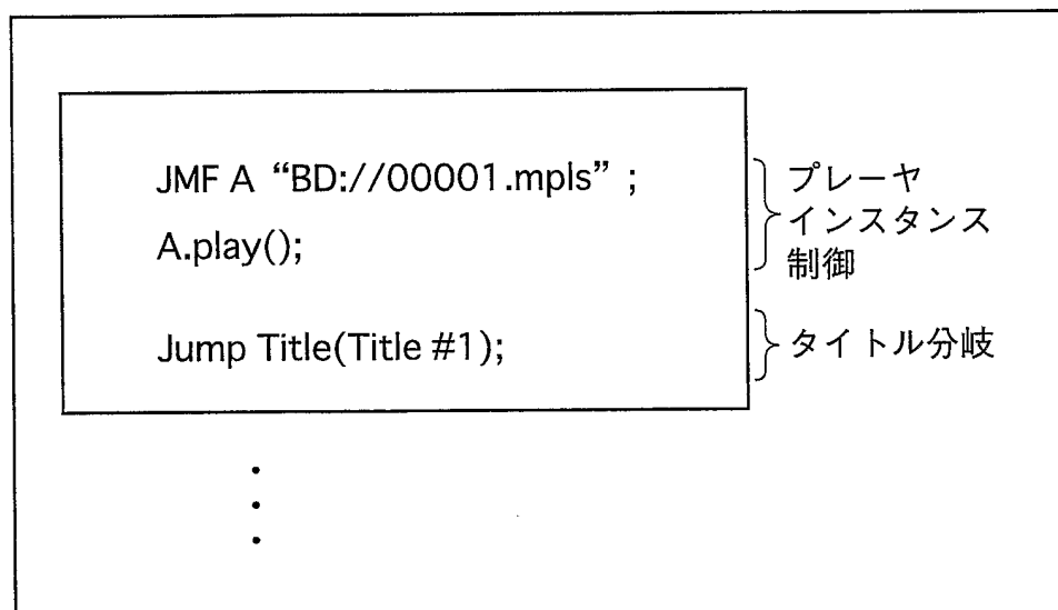
(b) xlet プログラム
