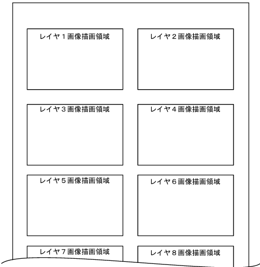
VRAMの内容
