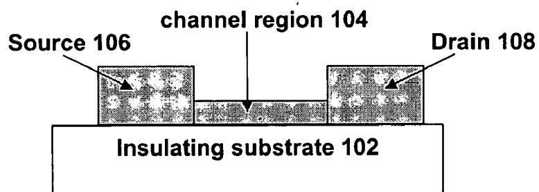
FIG. 8C (X-X view)
