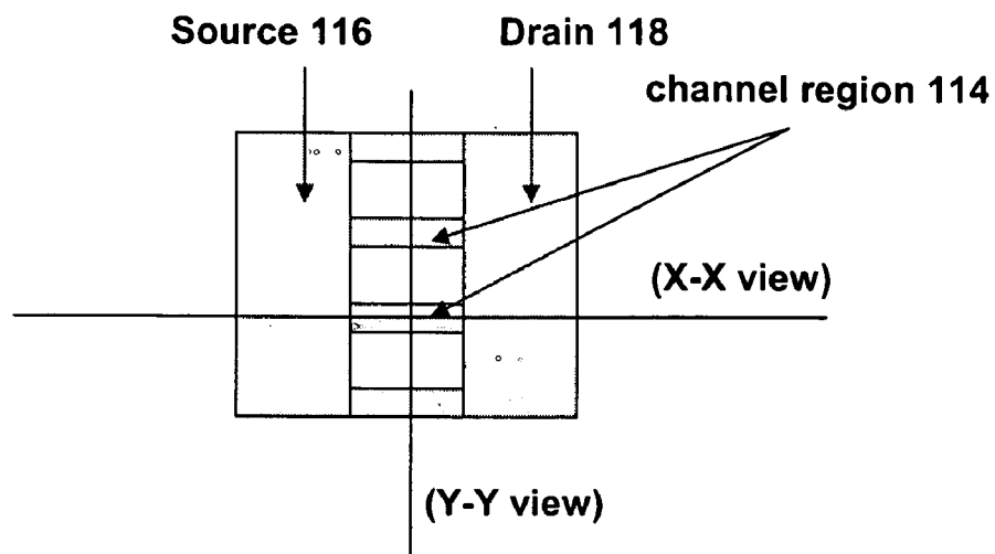
FIG. 9A (top view)
