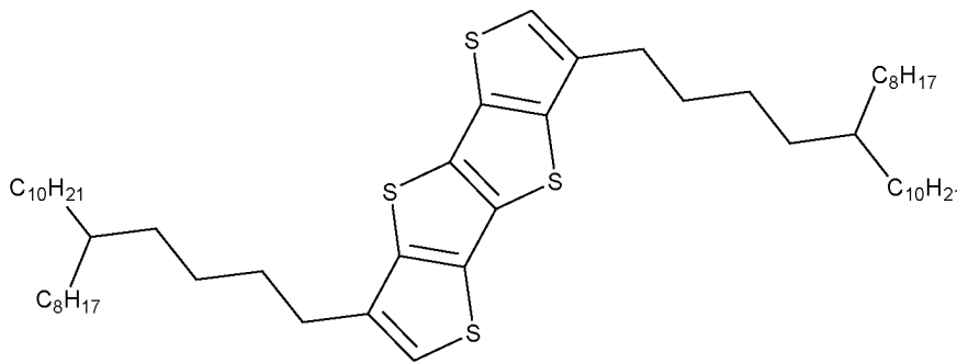
DC5BC8C10FT4
