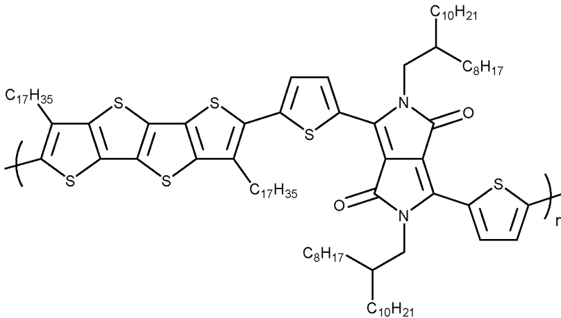
PTDC2BC8C10DPPTDC17FT4
