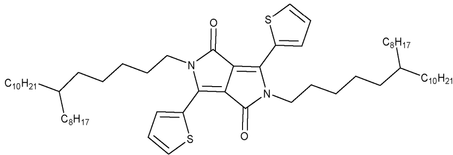
DTDC6BC8C10DPP
