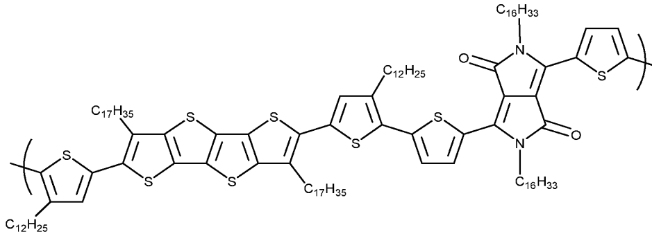
PC12(o)TTDC16DPPTC12(o)TDC17FT4
