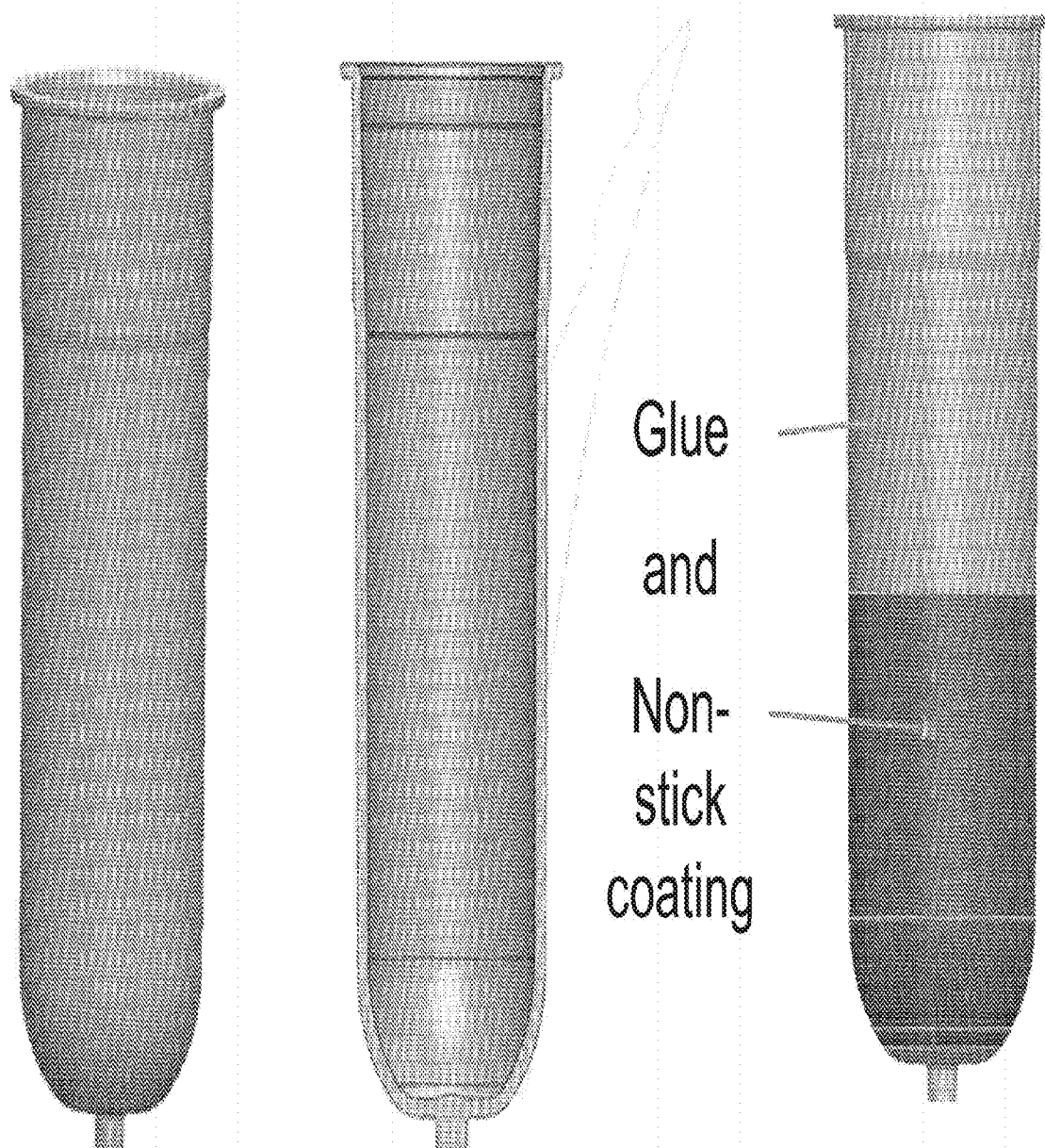
Fig. 21 - Piston Flair Inside Layer
