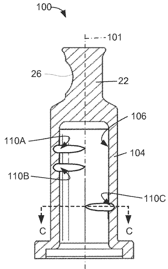
section B-B FIG. 2B
