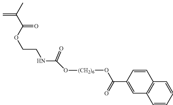
MONOMER (1)
