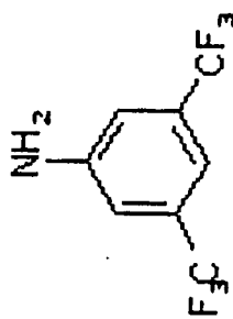
3,5-Bis(trifluoromethyl)aniline
