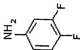
3,4-Difluoroaniline
