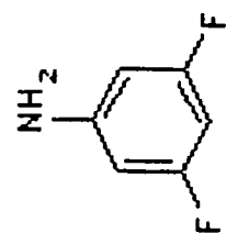
3,5-Difluoroaniline
