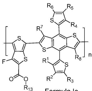
Formula Ic
