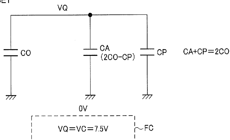
FIG. 4B MAXIMUM DATA VOLTAGE
