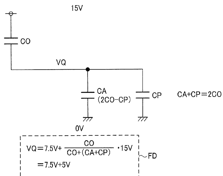
FIG. 4B MAXIMUM DATA VOLTAGE
