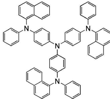
1'-TNATA
