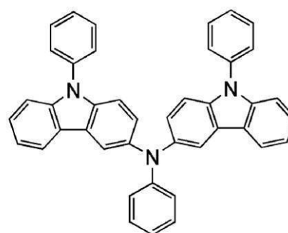
PCzPCA1
