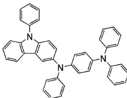
PCzDPA1
