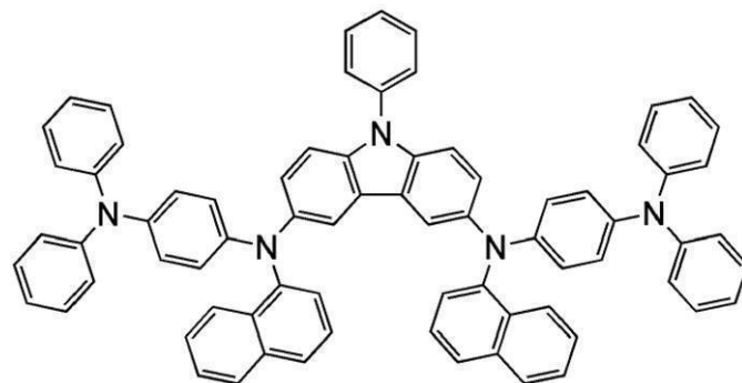
PCzTPN2
