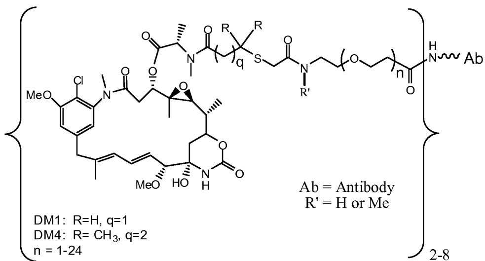
Ab-PEG-SIA-DM1/DM4
