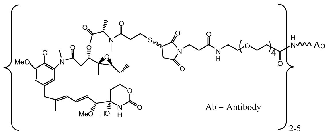
Ab-PEG4-Mal-DM1
