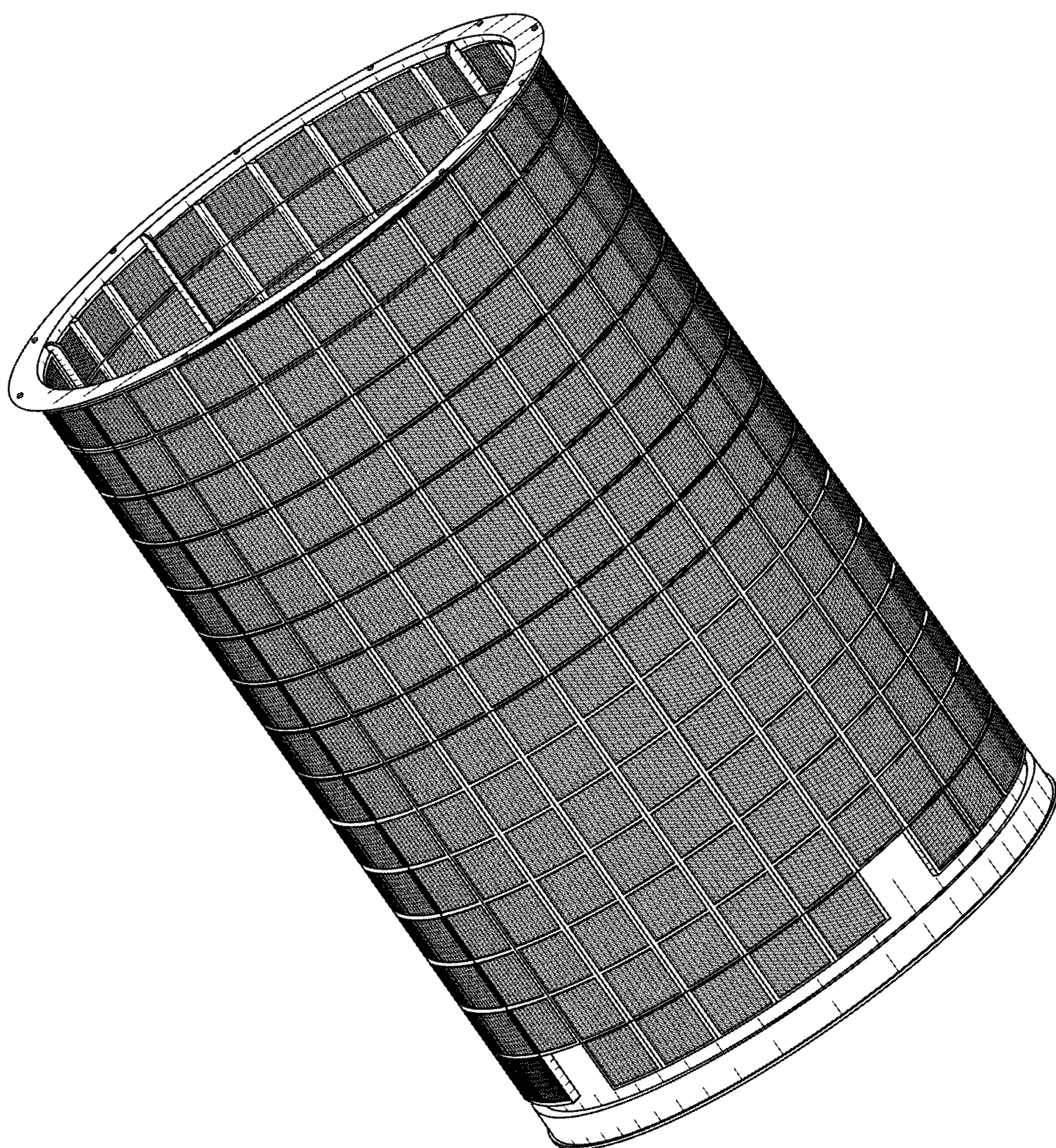
【立體圖】
