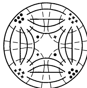
TM_{210} Fig. 1C
