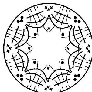
TM_{410} Fig. 1F
