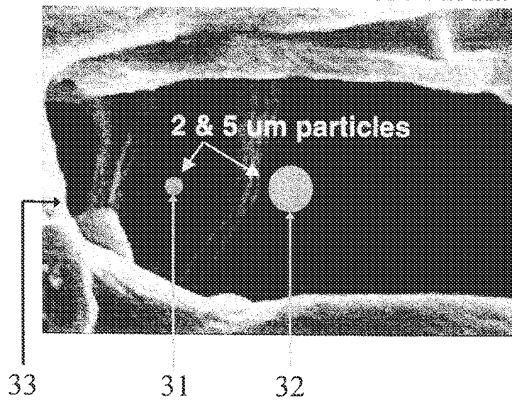
FIG. 3A Cellulose Media
