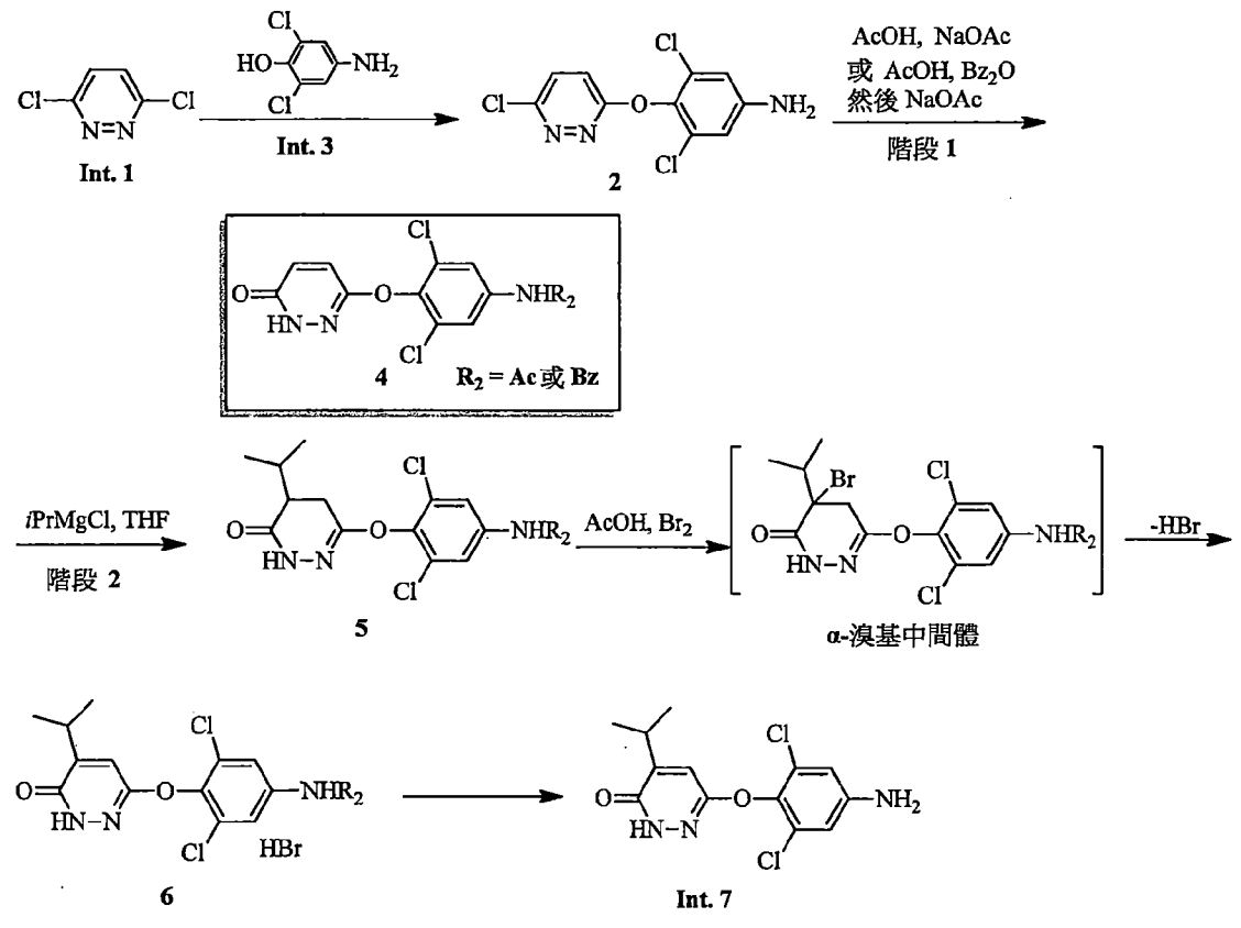
反應圖 1
