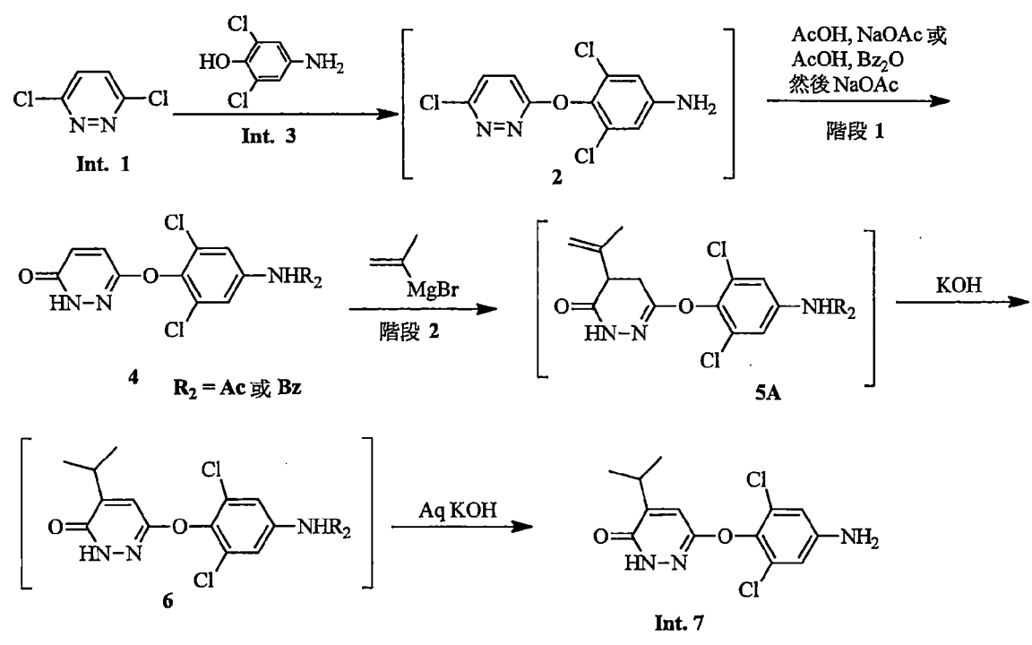
反應圖 2
