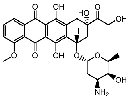
doxorubicin
