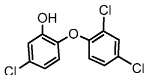
triclosan
