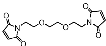
BM(PEG) 2
