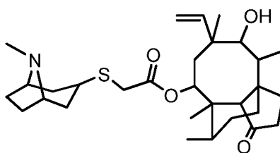
retapamulin
