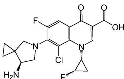
sitafloxacin
