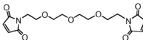
BM(PEG) 3
