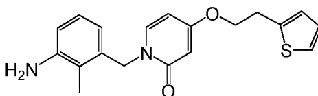
CG-400549
