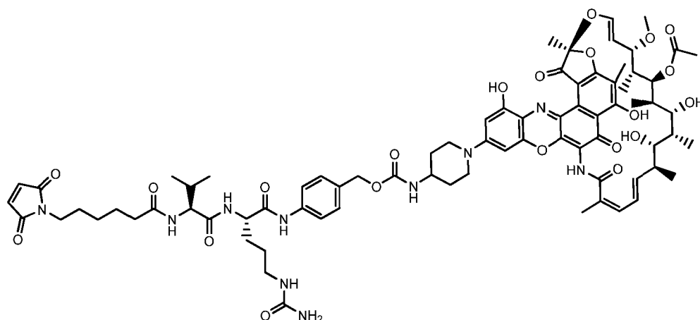
MC-vc-PABC-(pipBOR)
