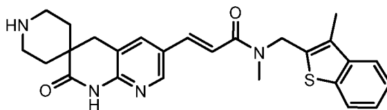
naphthyridone
