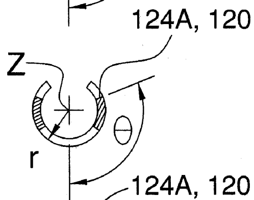
FIG. 6D SECTION G-G
