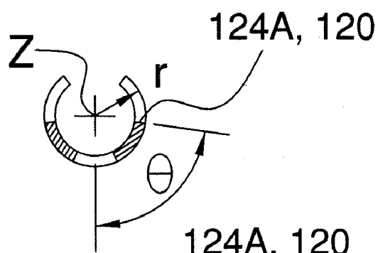
FIG. 6E SECTION H-H
