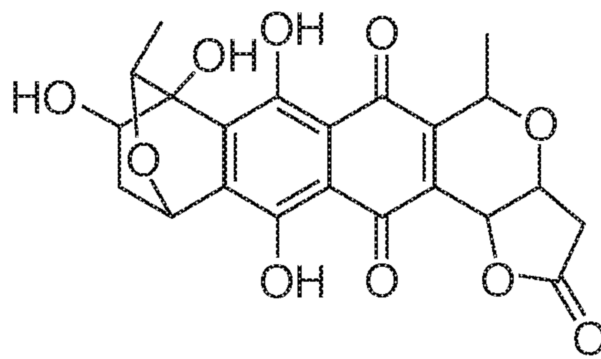
(2) Granaticin A
