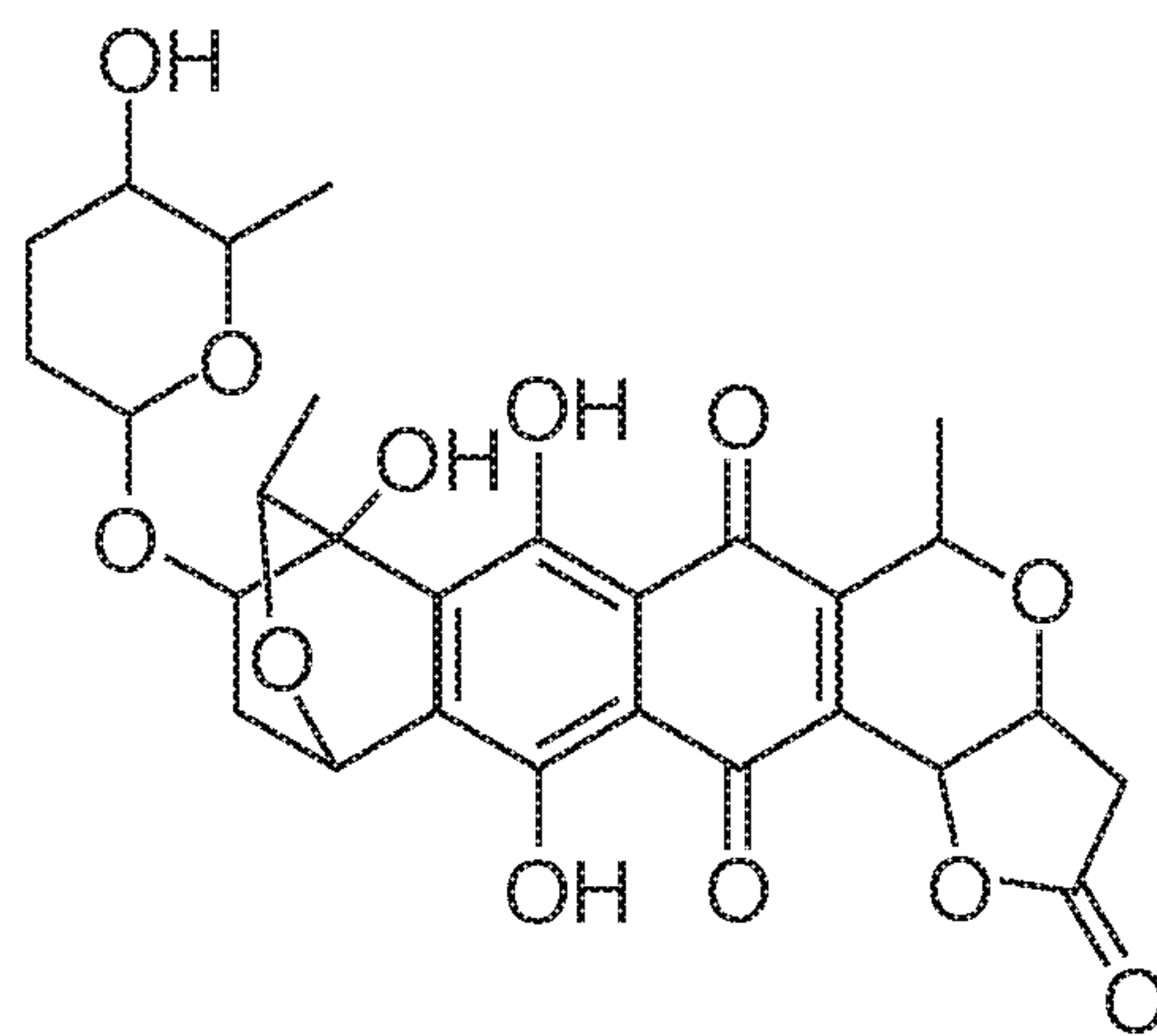
(1) Granaticin B
