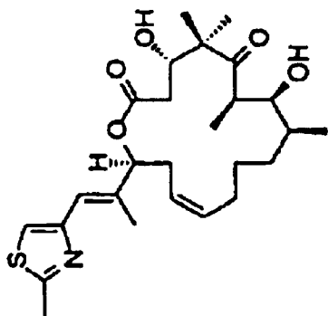
desoxyepothilone A
