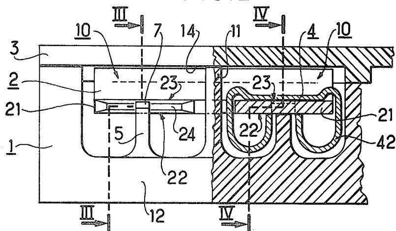
2/2 FIG. 2
