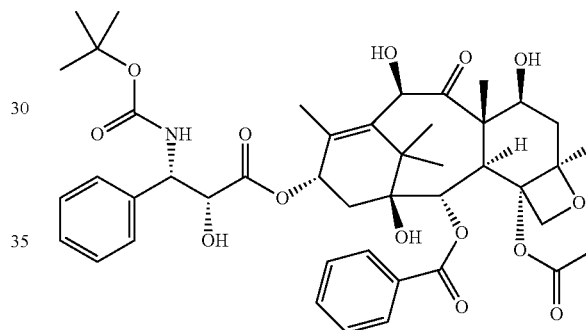
docetaxel
