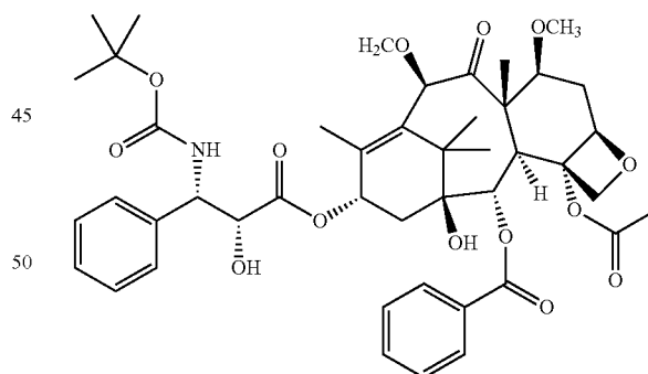
cabazitaxel
