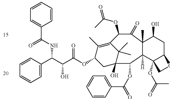
paclitaxel
