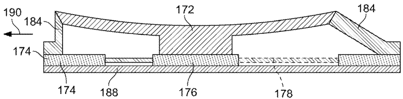
FIG. 13C
