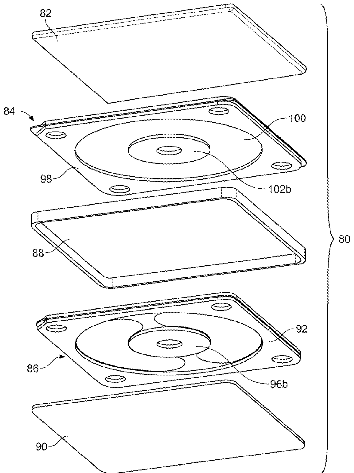
FIG. 9B
