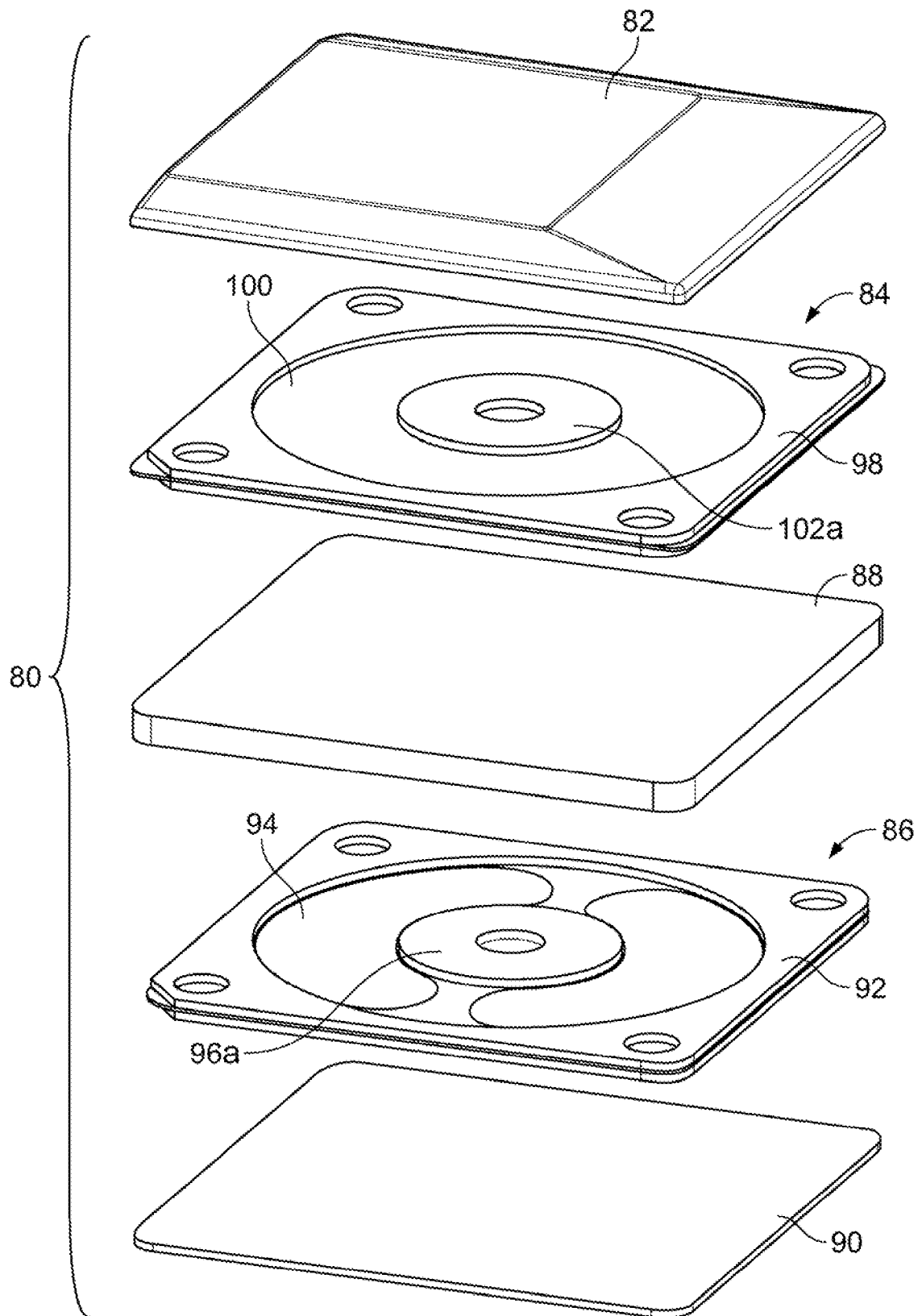
FIG. 9A
