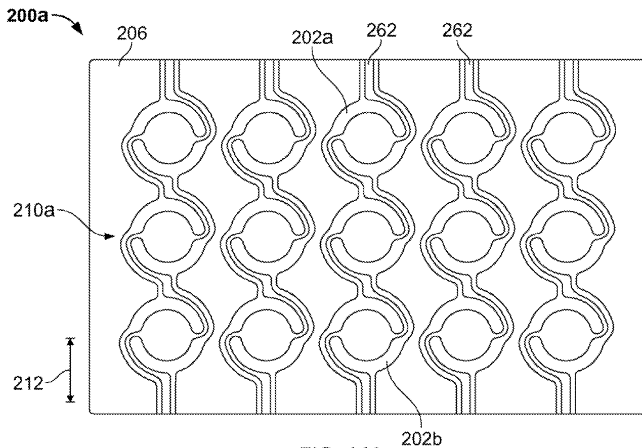
FIG. 14A
