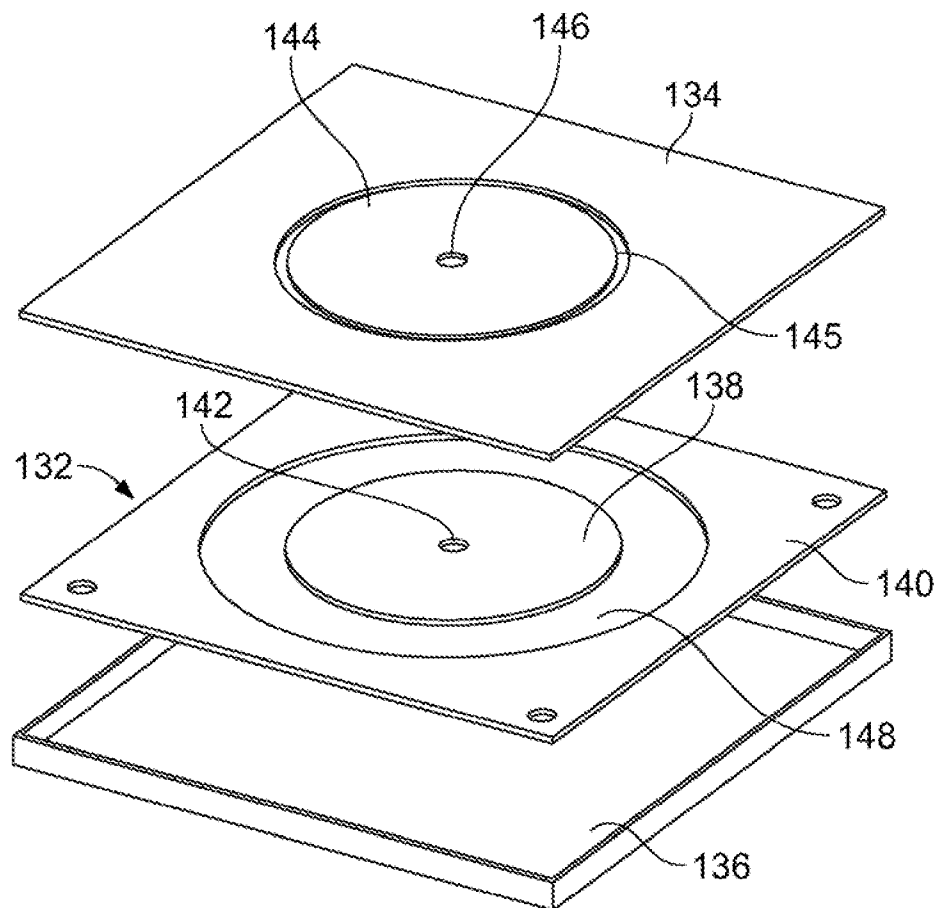
FIG. 11B
