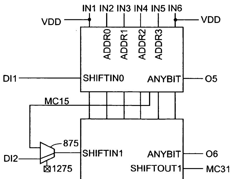
FIG. 13 (16x2 SRL)
