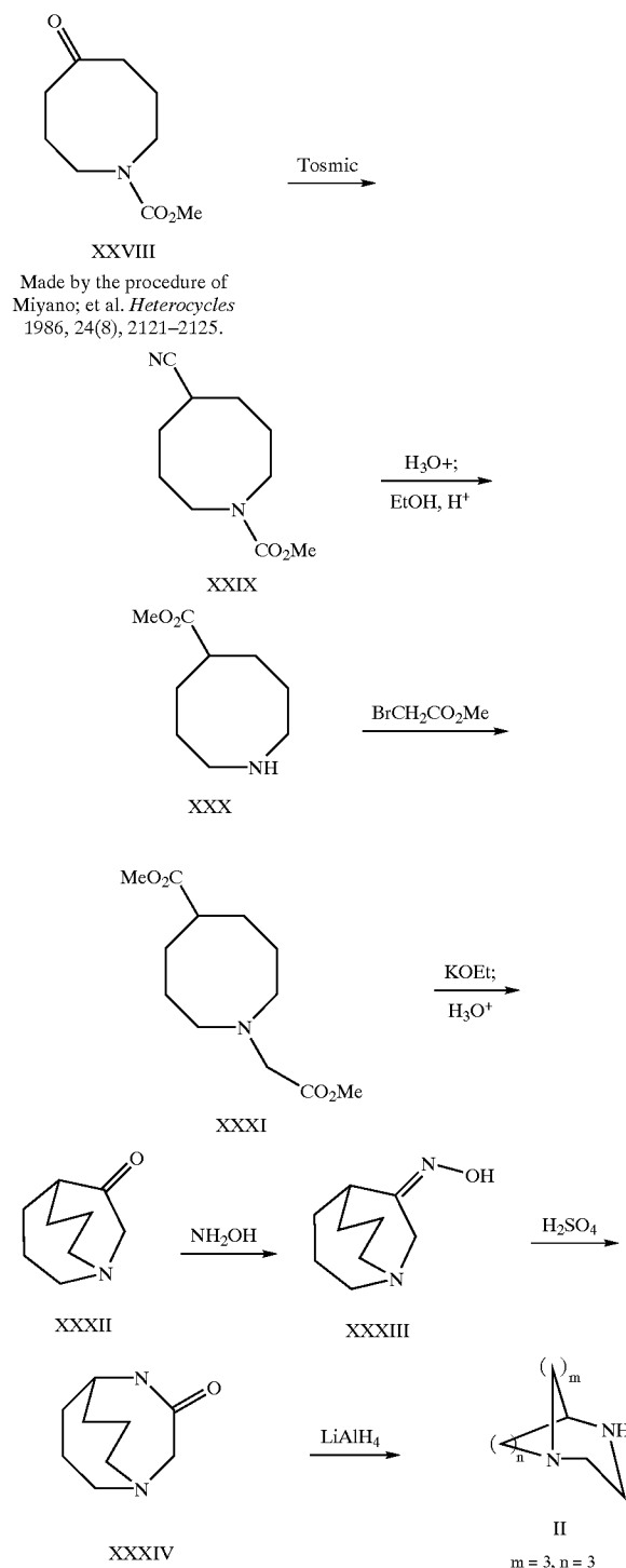
Schem VIII
