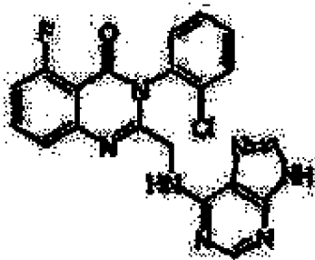
3-(2-хлорфеніл)-5-флуор-2-[(9H-пурин-6-іламіно)-метил]-3H-хіназолін-4-он (d-072)
