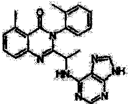
5-метил-2-[1-(9H-пурин-6-іламіно)етил]-3-о-толіл-Н-хіназолін-4-он (d-081)
