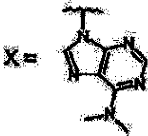
2-(6-диметиламінопурин-9-ілметил)-5-метил-3-о-толіл-3Н-хіназолін-4-он (d-082)
