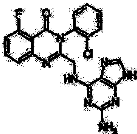
2-[(2-аміно-9H-пурин-6-іламіно)метил]-3-(2-хлорфеніл)-5-флуор-3H-хіназолін-4-он (d-074)
