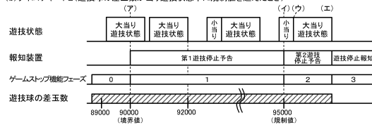
(c) タイムチャート3(遊技球の差玉数が当り遊技状態以外のときに規制値を超えたとき)
