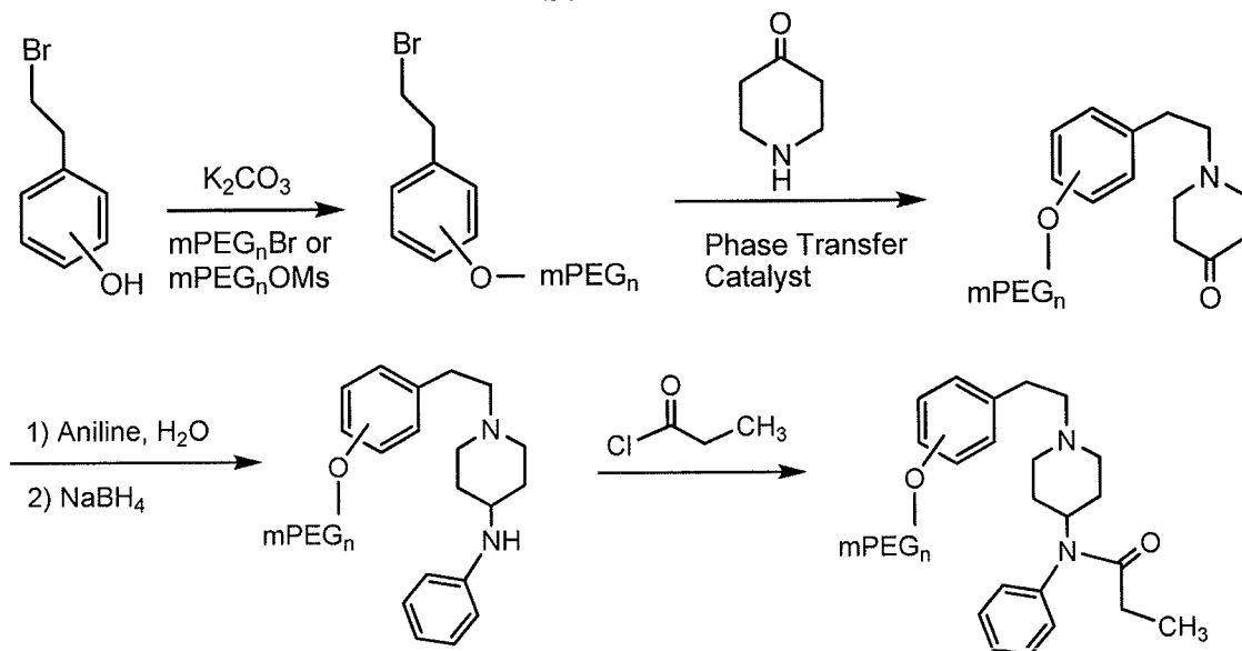
Scheme 4-A
