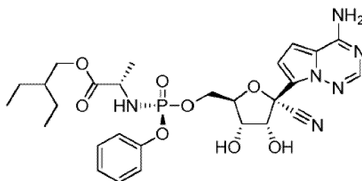
(Composé 1),
