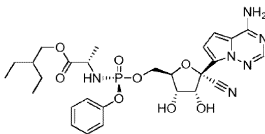
(Verbindung 1)
