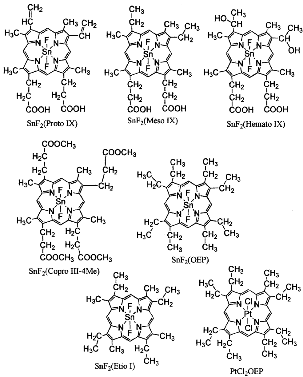
[化學式 1]
