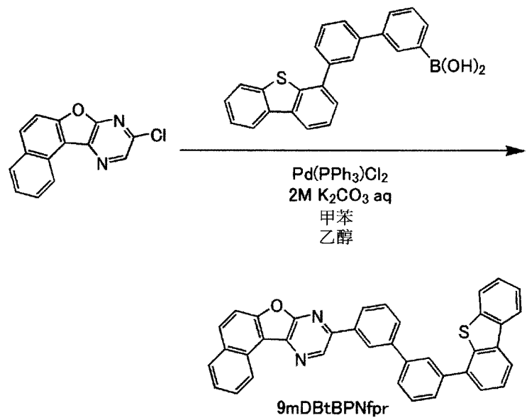
[化學式 16]
