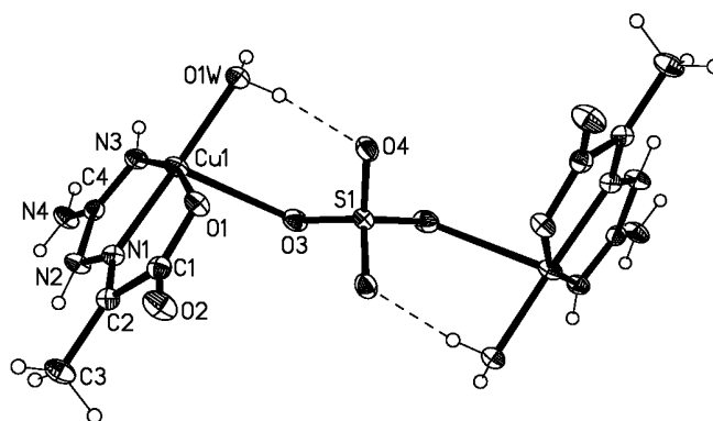
Fig. 2. Structura complexului [\text{Cu}_2\text{SO}_4 (\text{Hagpa})_2(\text{H}_2\text{O})_2]\cdot\text{DMSO} – \mu_2 -(sulfato)-bis(aqua-(aminoguanizonei acidului piruvic))-cupru(II) dimetilsulfoxid, (DMSO nu este prezentat, pentru a simplifica desenele)
