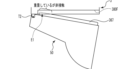
(B 3) 第2開状態 (開放角度: 約20度)
