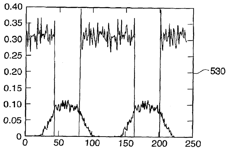
FIG. 5c 0.01 Torr
