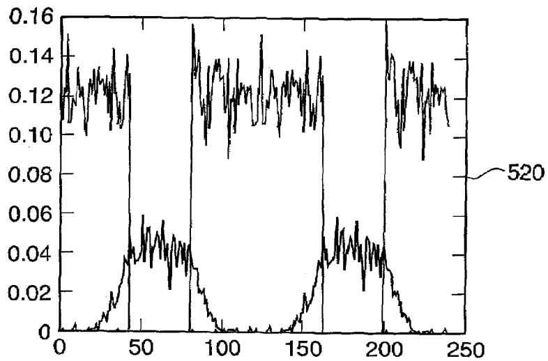
FIG. 5b 0.1 Torr
