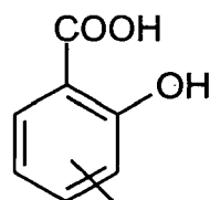
Salicylsäurerest
