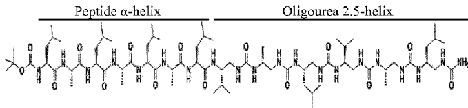
oligomer 7
