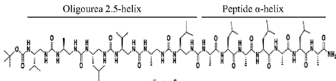
oligomer 8
