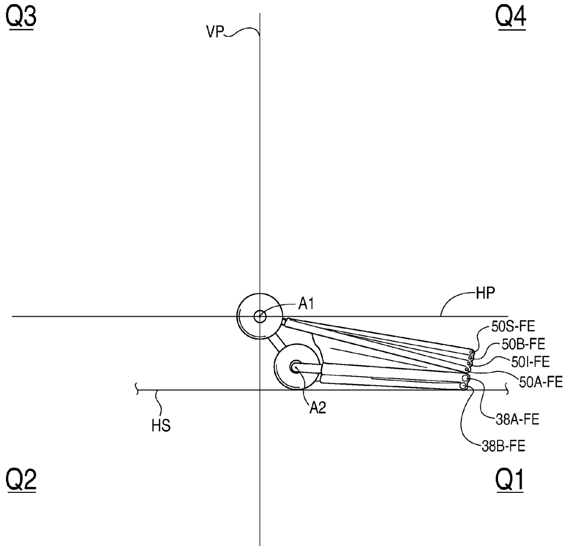
FIG. 21A
