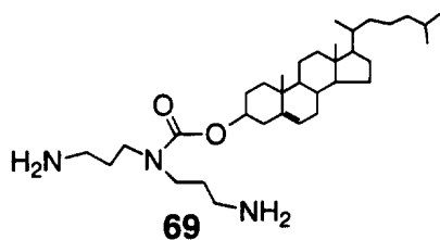
69 N,N bis (3-aminopropyl) cholesteryl carbamate
