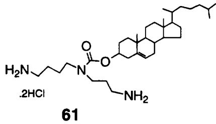
61 N 4 -spermidine cholesteryl carbamate di HCl salt
