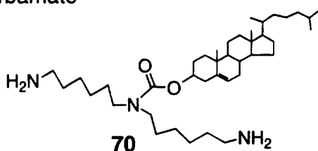
70 N,N bis (6-aminohexyl) cholesteryl carbamate
