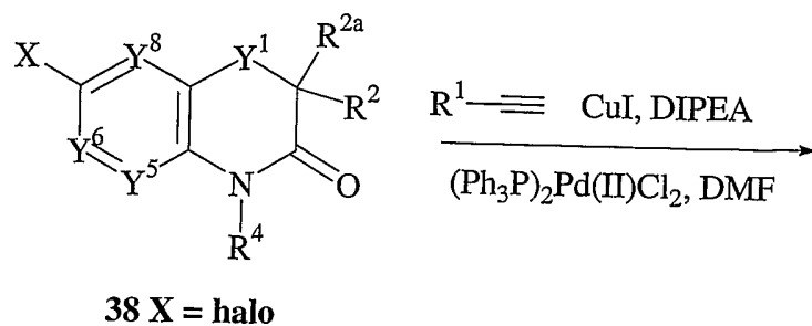
Scheme 5a.
