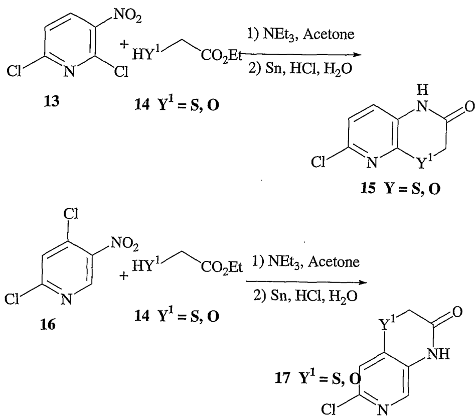
Scheme 3a.
